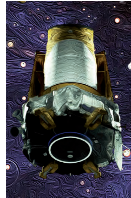
Das Weltraumteleskop „Kepler“ suchte von 2009 bis 2018 nach erdähnlichen Planeten.
