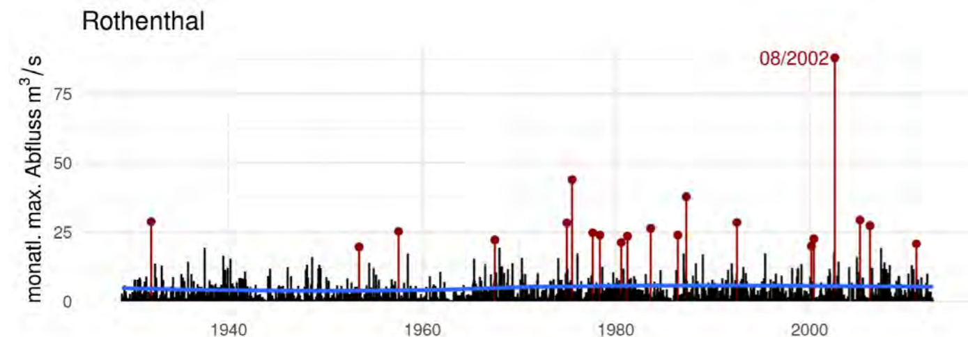
Monatliche Maxima des Abflusses am Pegel Rothenthal an der Natzsung im Flussgebiet der Mulde in Sachsen: Hervorgehoben sind alle Werte, die größer sind als das 98%-Quantil dieser Monatsmaxima. Solche Extremereignisse häufen sich in der zweiten Hälfte des Beobachtungszeitraums ab den späten 1970er-Jahren. Dies gilt auch für viele andere Pegel in Sachsen. Der blau eingezeichnete, zeitvariabel geschätzte Mittelwert ist hingegen recht stabil. Als Jahrhundertereignis kann der größte beobachtete Wert im August 2002 gelten: Dieser ist in etwa doppelt so groß wie der zweitgrößte Wert. Die anderen Extremwerte liegen hingegen in einer ähnlichen Größenordnung.
