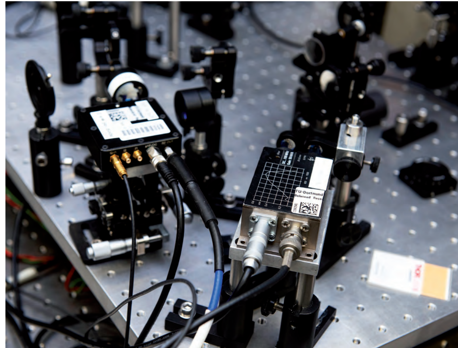
Der Winkel, um den sich die Polarisation des Laserstrahls dreht, wird mit sogenannten balancierten Foto-Dioden gemessen. Davon gibt es verschiedene Modelle: Die Diode vorne rechts ist sensitiver, aber dafür langsamer und deckt einen kleineren Frequenzbereich ab (bis 100 Megahertz). Die linke Diode kann schnellere Messungen in einem breiteren Frequenzspektrum vornehmen, ist dafür aber weniger sensitiv (bis 1000 Megahertz).
