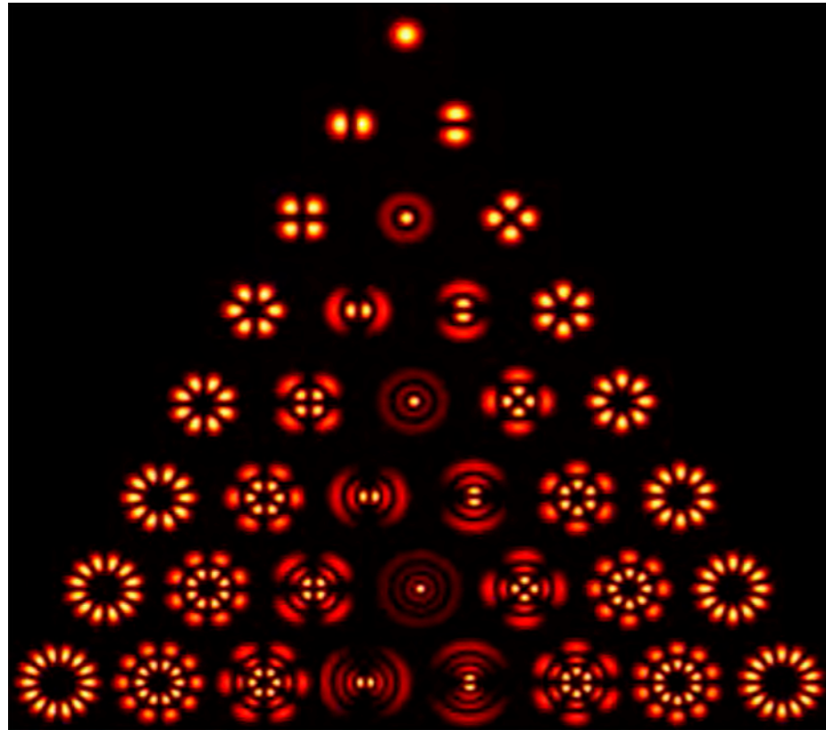
Für die Lichtwellen in Glasfasern gibt es verschiedene Lösungen der Wellengleichung, Moden genannt.
