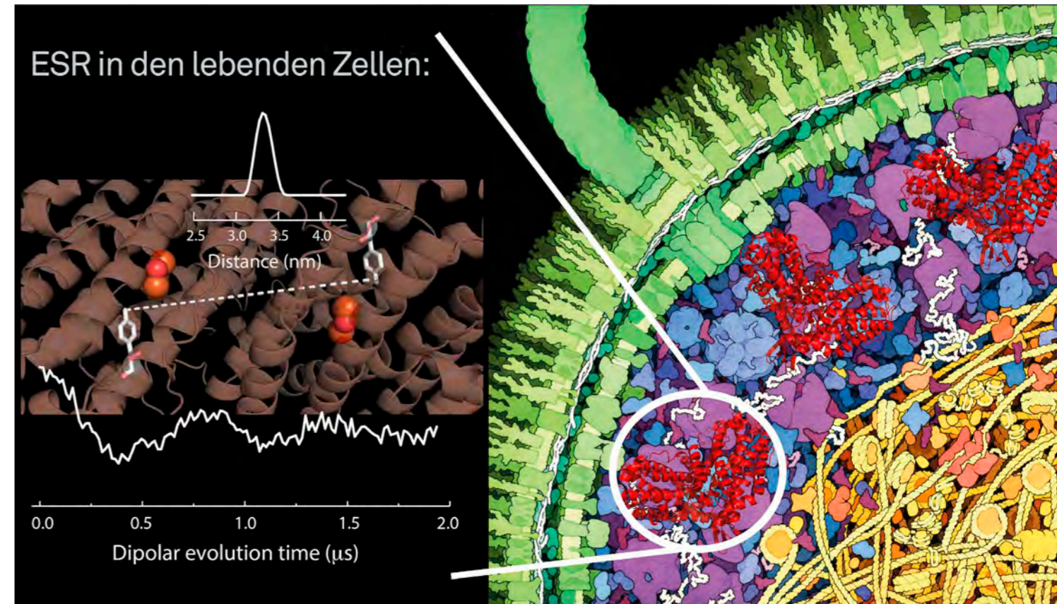
Mit Hilfe von ESR-Spektroskopie kann Kasanmascheff Proteine wie die Ribonucleotid-Reduktase in lebenden Zellen beobachten. (Quelle: David Goodsell/ Collage Müge Kasanmascheff)
